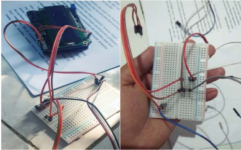
Gambar 3.8 Rangkaian Kontrol LCD 16X2 Keypad dengan papan Breadboard
