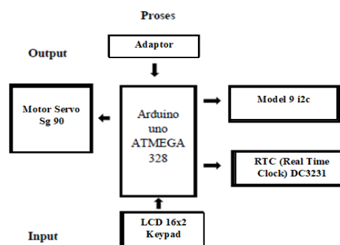
Gambar 3.1 Diagram Blok Sistem
